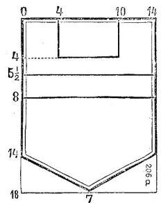
2a. Schnittübersicht zu Abb. 2.
