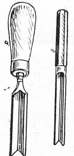
5. Geißfuß. 5a. Dreieckseisen.
