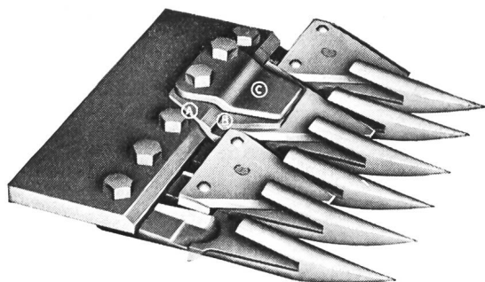
Bild: Die patentierte Messerführung
