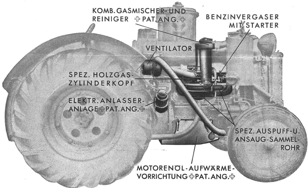
Einbau von Ford 4 Zyl. Motoren auf Vevey-Diesel
