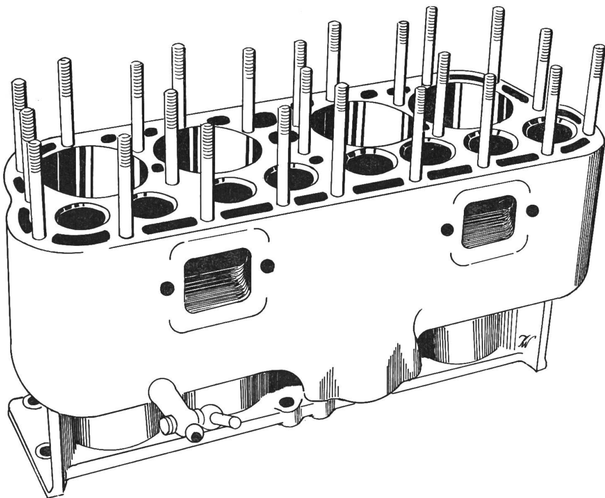
Fig. 77: Zylinderblock eines älteren 4-zylindrigen Benzinmotors. Die vielen Schraubenbolzen sind nötig, damit eine einwandfreie Abdichtung der einzelnen Verbrennungsräume möglich ist. Heute wird dieser Teil meist mit dem Kurbelgehäuseoberteil zusammengegossen.
