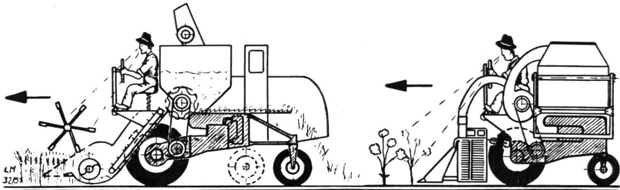
Abb. 9: Optimale Anordnung von Front-Mähwerk oder -Pflücker zum Einmann-Bediener bei USA-Grosslandmaschinen (JHC SP 127, Cotton Picker M 11 H).
