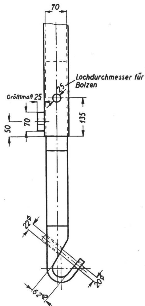
Abb. 5: DIN 9672 — Ackerschlepper, Schwingrahmen mit Kupplungshaken
