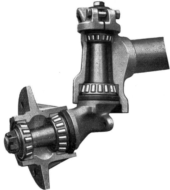
Detail mit Schräggrollenlager der Radgelenke am Achsschenkel. Die Schräggrollenlager können leicht nachgestellt werden. Das lästige Spiel der Vorderräder wird dadurch behoben.
