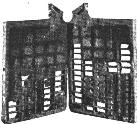
Abb. 2: Durch Erschütterungen (infolge unzweckmässiger Befestigung) wurde die aktive Masse aus den Gittern losgeschüttelt.
