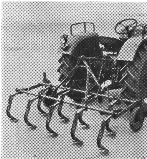
Kultivator mit 9 abgefederten Zinken
