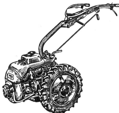
AGRIA-Universal Type 1700, 6—7 PS, mit 6-Gang-Getriebe, 2 Zapfwellen, beidseitigen Innenbackenbremsen, beidseitigen Triebbradkupplungen, 4 Spurbreiten. Preis mit Stufenabstufen u. Pneurädern, 4,50x14 AS Fr. 2430.-.
