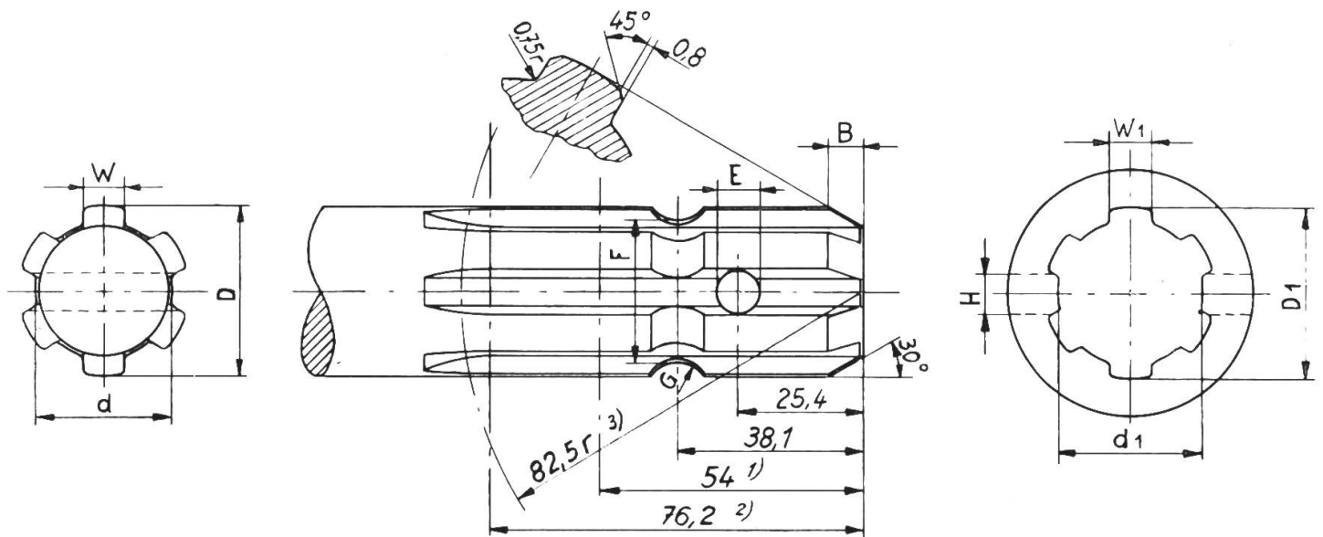
Abb. 3: Abmessungen der von der ISO vorgeschlagenen Zapfwelle. (Masse in mm)
