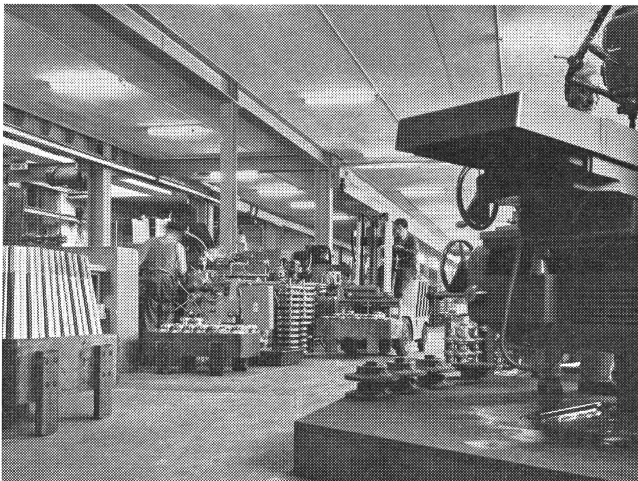
Teil-Ansicht des neuen Werkzeugmaschinenparkes, bestimmt zur Serien-Fabrikation der Traktoren
