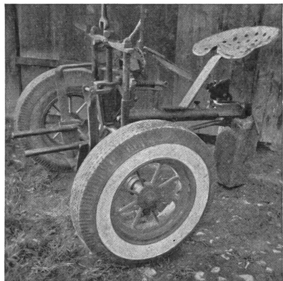
Abb. 1b: Der Geräteträger der Spinne
