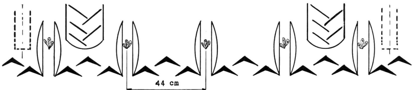
Abb. 5: Bei der Spurweite des Traktors von 130 cm (genau 132 cm) und 44 cm Reihenabstand kommen die Säscharen zwischen die Radspuren des Traktors und der Sämaschine zu liegen.
