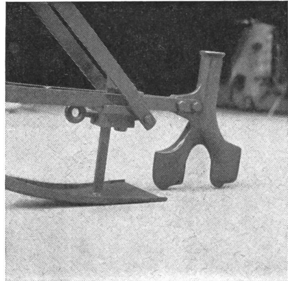
Abb. 4b: Doppelsächar mit Gleitkufe.
