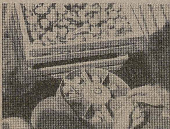
Patent-Setzautomat mit 8-teiligem Zellenrad beim Setzen von vorgekeimten Kartoffeln.
