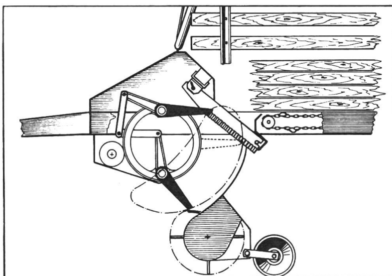
Funktion der Doppelschwinge am Ladewagen HAGEDORN Typ LD mit Schneidwerk (Scherenschnitt)
