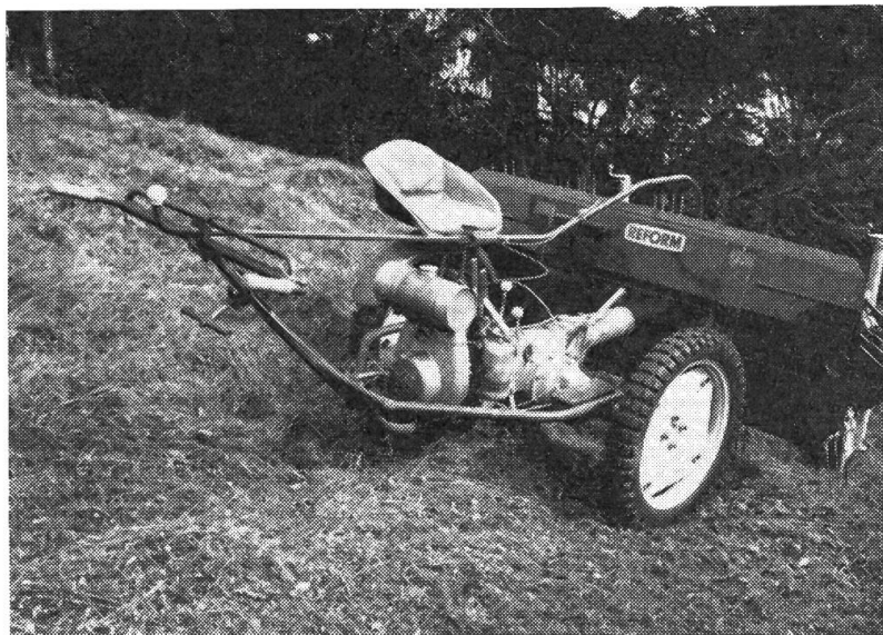
Abb. 4: Ein Heuer mit quer zur Fahrtrichtung montiertem Sitz und Stützradlenkung
