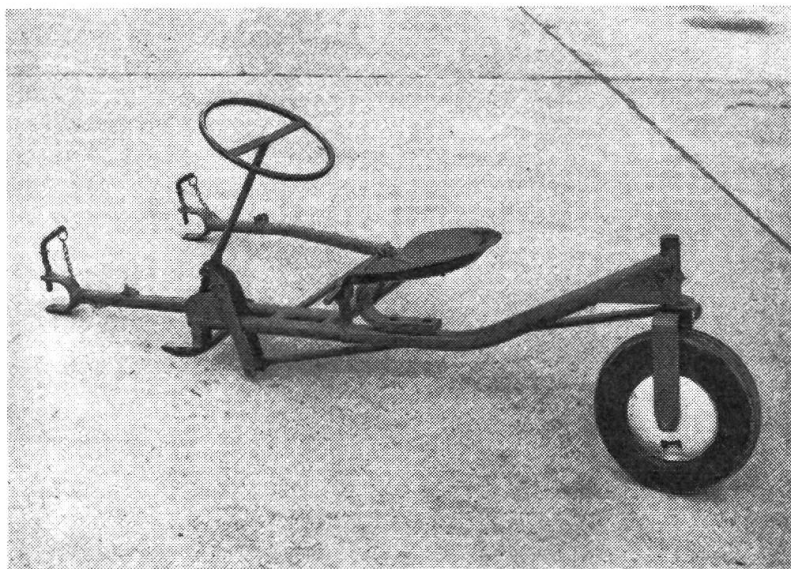
Abb. 3: Der Nachlaufsitz als Zusatzausrüstung bietet dem Bedienungs- mann Arbeitserleichterung
