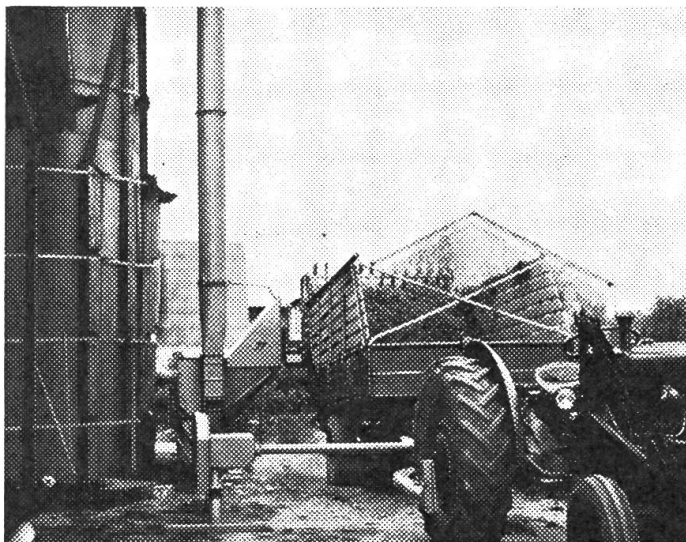
Das «JF»-SILOWURFGEBLÄSE (Zapfwellenantrieb) und der «JF»-Allzweckwagen (als Häckselwagen) mit dem Kombi- und Seitenabblader beim Füllen des Silo.
