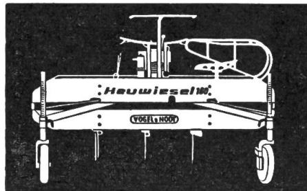
Kombigerät Heuwiesel zum Heuen, Mähen und Düngerstreuen. 7,5 PS, Arbeitsbreite 1,60 m.
