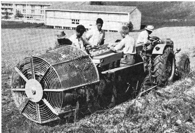
Abb. 2: Siebtrommel- Sammelgraber
