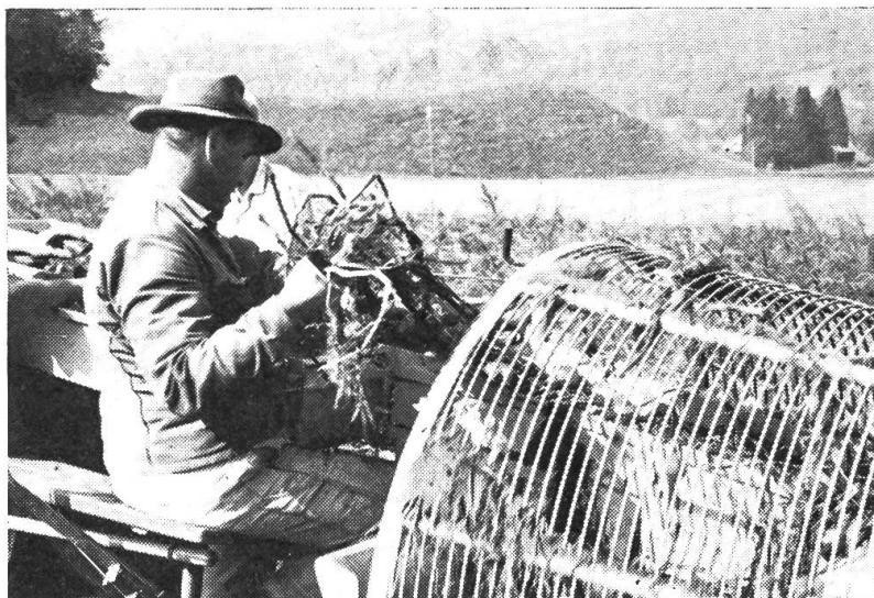
Abb. 9: Beim Siebtrommel-Sammelgraber müssen die Stauden von Hand herausgelesen werden.
