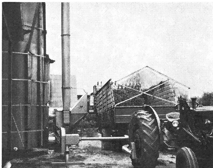
Das «JF»-SIELOWURFGEBLÄSE (Zapfwellenantrieb) und der «JF»-Allzweckwagen (als Häckselwagen) mit dem Kombi- und Seitenabladern beim Füllen des Silo.
