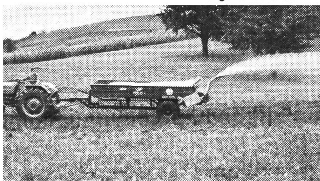
Der «JF»-ALLZWECKWAGEN als Saug- und Druckfaß beim Güllen (12 m Streubreite). Der Antrieb der Zentrifugal- und Füllpumpe erfolgt über die Zapfwelle.
