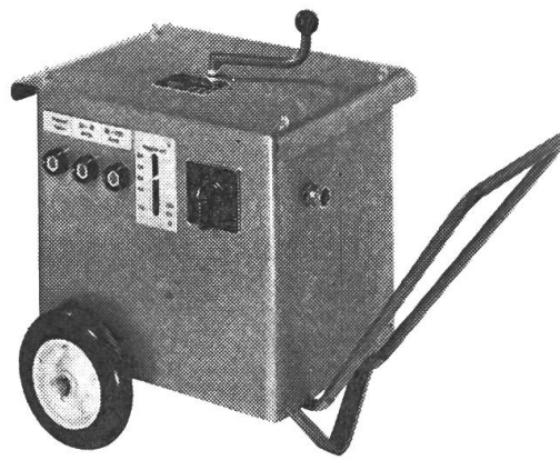
Typ Industrie 30–200 Amp. stufenlos, 380 V, 85 kg. Fr. 980.— + Schweiss- platzausrüstung
