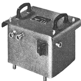
Typ Knirps Für Bastler 2 Stufen, 220 V, 25 kg. Fr. 350.— + Schweiss- platzausrüstung
