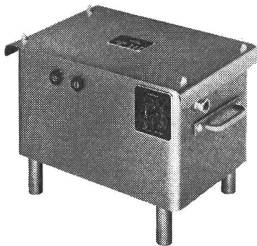
Typ Schweissboy-Super 30–150 Amp. 5 Stufen, 380 V, 68 kg. Fr. 700.— + Schweiss- platzausrüstung
