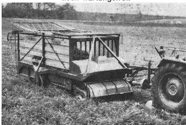
Der LADEWAGEN KADETT beim Eingrasen. Mähen und Aufladen gleichzeitig. Kraftbedarf ab 12 PS. Der ideale Wagen für Fuderaufzug.
