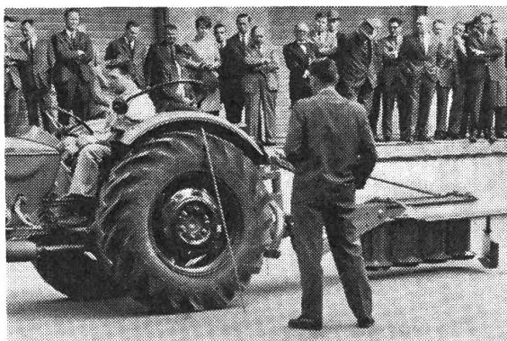
Vorführung des nach dem holländischen System Zweegers konstruierten Kreiselmäähers KM mit vier Trommeln. Arbeitsbreite 1,60 m. (Werkphotos Fahr)
