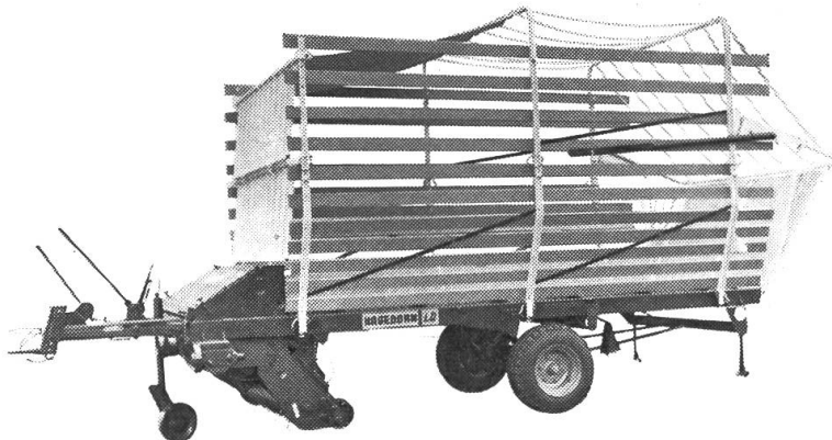
Ladewagen HAGEDORN «LD»
