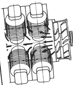
Luftkühlung, zwangsläufige Motorölkühlung
