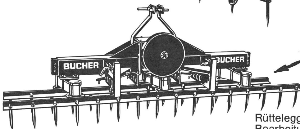
Zinkenegge zwei- und dreifeldrig mit Spurlockerern.
