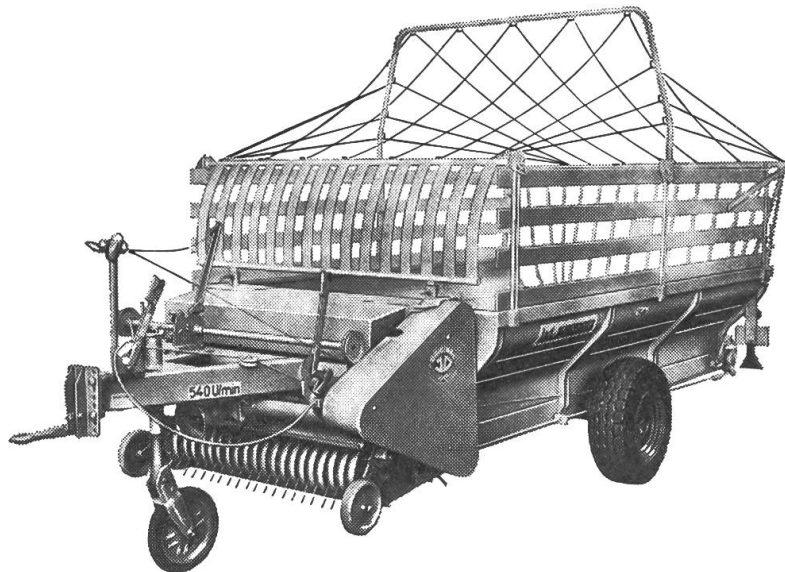
Das ist der LELY-DECHENTREITER-Ladewagen, Typ LW 2 K
