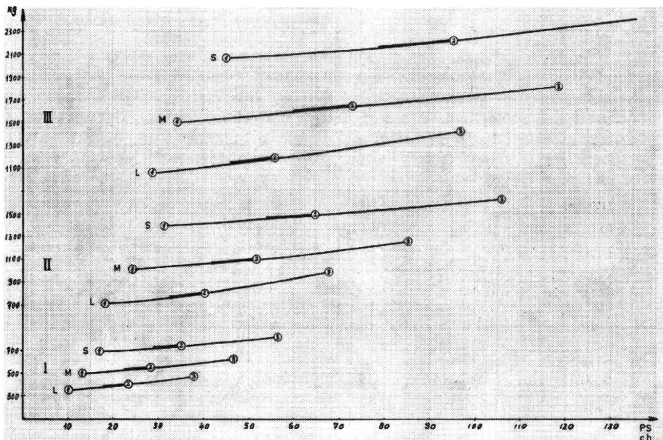
Abb. 8: Zug- und Motorleistungsbedarf je nach Pfluggrösse, Bodenart und Fahrgeschwindigkeit.
