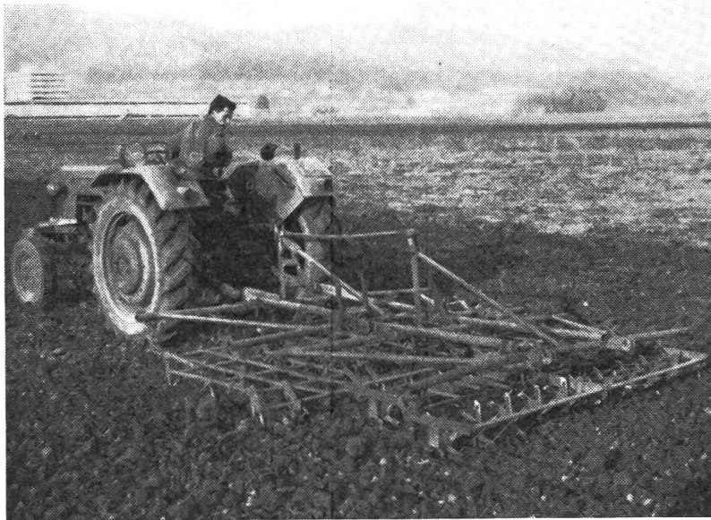
Abb. 18: Eine Gerätekombination, bestehend aus einer Löfflegge und einem Krümmer (Drahtwalze), eignet sich sehr gut für die Saatbettvorbereitung für Zuckerrüben.
