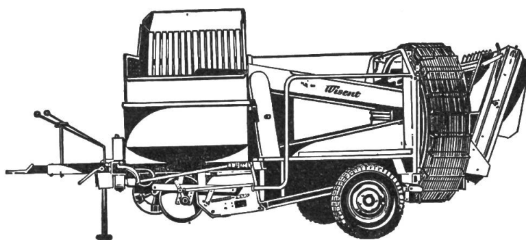
Typ RB-68 mit grossem Bunker von ca. 1500 kg Fassungs- vermögen (Normalbunker ca. 1100 kg Inhalt), Kippen vollhydraulisch.
