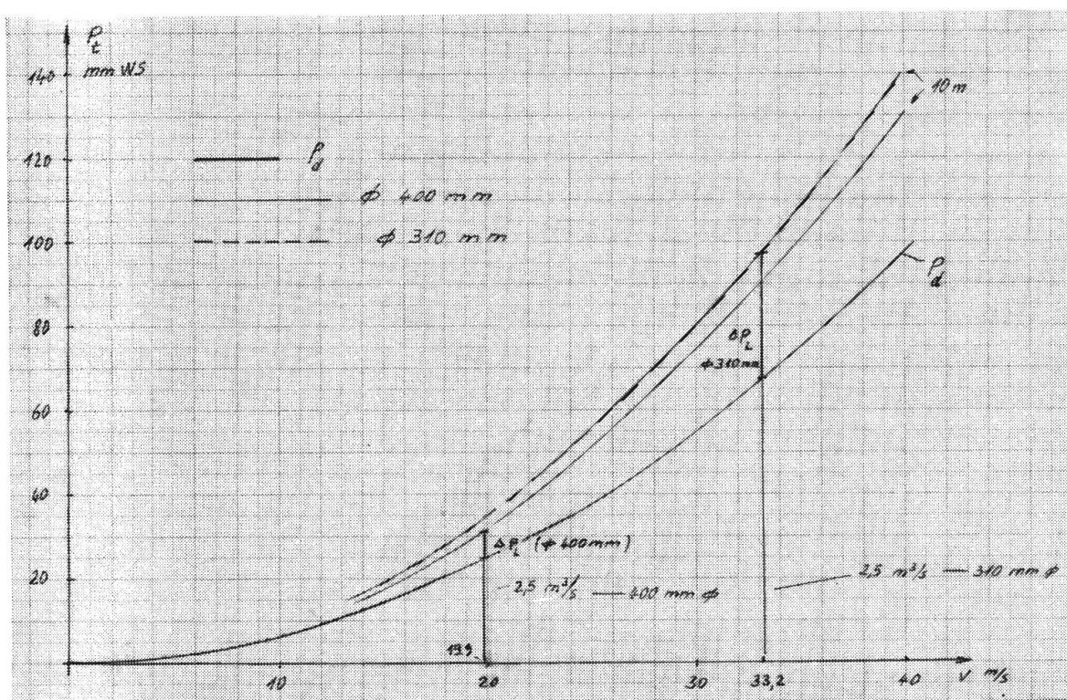
Abb. 6: Widerstandsparabel für Rohrleitungen mit 400 mm Durchmesser und 310 mm Durchmesser bei 10 m Rohrlänge. Annahme: Luftfördermenge 2,5 \text{ m}^3/\text{s} ; Ergebnis für Rohr mit 400 mm Durchmesser: Luftgeschwindigkeit 19,9 \text{ m/s} , Betriebsdruck 32,7 \text{ mm WS} ; für Rohr mit 310 mm Durchmesser: Luftgeschwindigkeit 33,2 \text{ m/s} , Betriebsdruck 97,6 \text{ mm WS} . P_d = dynamischer Druck, \Delta P_L = Rohrreibungsverlust.
