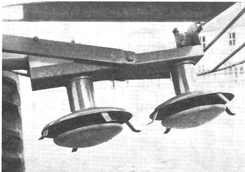
Abb 2: Der neue «Bamlett»- Kreismäher mit Oben- antrieb und Laufteiler.
