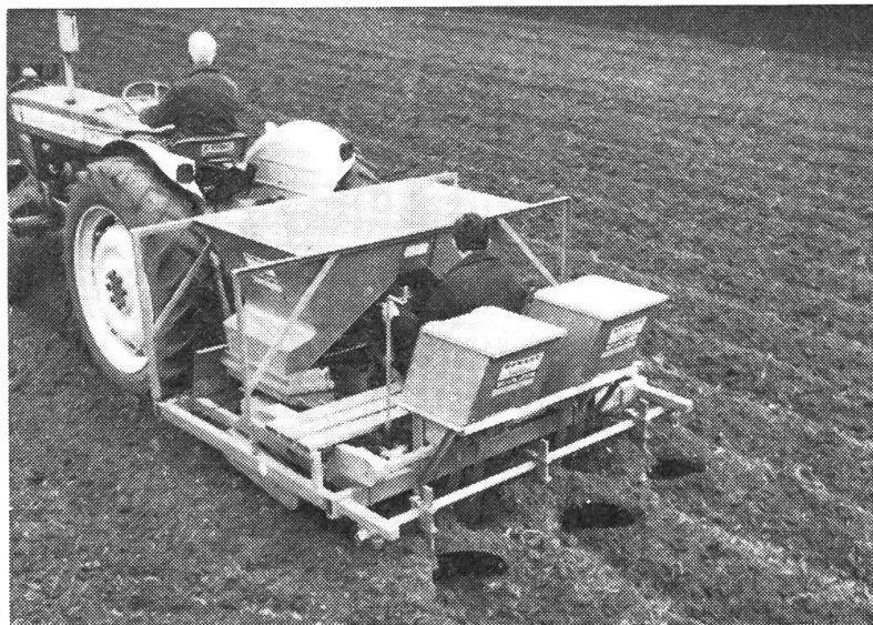
Abb. 3: «Howard» Hochleistungs- Kartoffellegemaschine für vorgekeimtes Pflanzgut mit Reihen- düngerstreuer.
