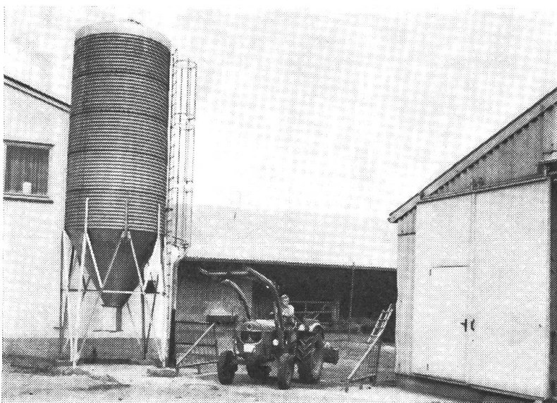
Abb. 3: Ausfahrt vom Offenlaufstall. Der Traktor fährt im Moment über einen Tretrost. Links erkennt man das Milchhaus und einen Siloturm für Kraftfutter. Im Hintergrund erkennt man ferner die überdachte Liegefläche des Offenstalles und rechts den überdachten Fressplatz. Dazwischen liegt der nicht überdachte Laufhof.
