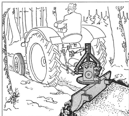
WIRA-Kehrmaschine für Traktoranbau.
