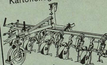
Rübenhacke
