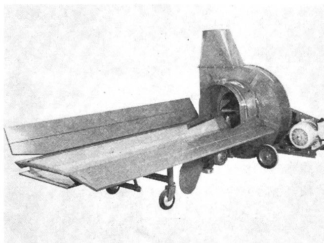
Abb. 1: Vielzweckfördergebläse mit Zubringerband.
