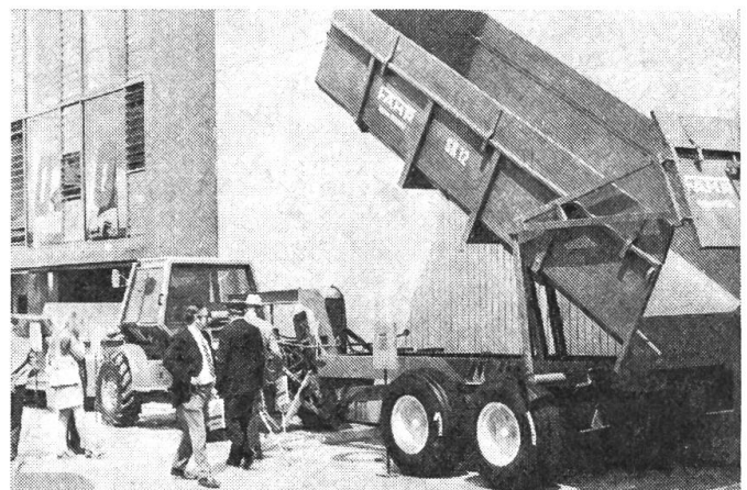
Abb. 2: Kippwagen aufgesattelt auf Grossgeräteträger (Deutz).
