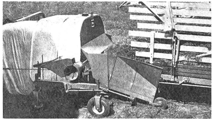
Abb. 6a: Silopresse an der Arbeit.
