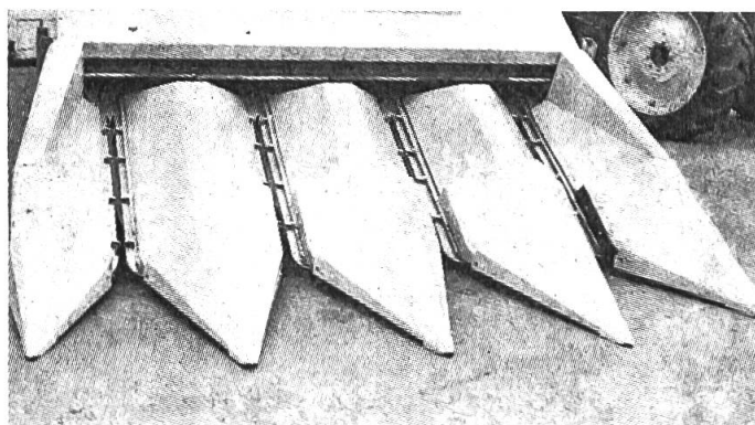
Abb. 9a: Vierreihiger Pflückvorsatz. Die Maisstengel werden von den Ketten nach hinten gefördert. . .
