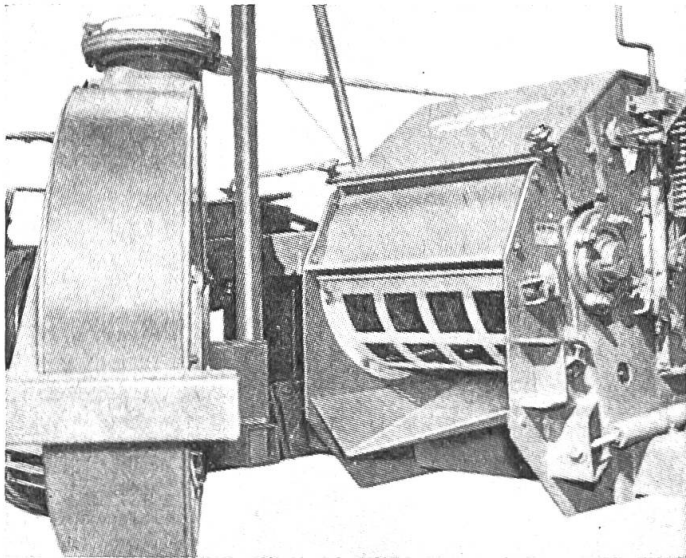
Abb. 4: Recuttereinsatz (Nachschneidevorrichtung an Trommelhäcksler) mit quadratischen Oeffnungen. Das Gebläsegehäuse lässt sich zum Auswechseln nach der Seite schwenken.
