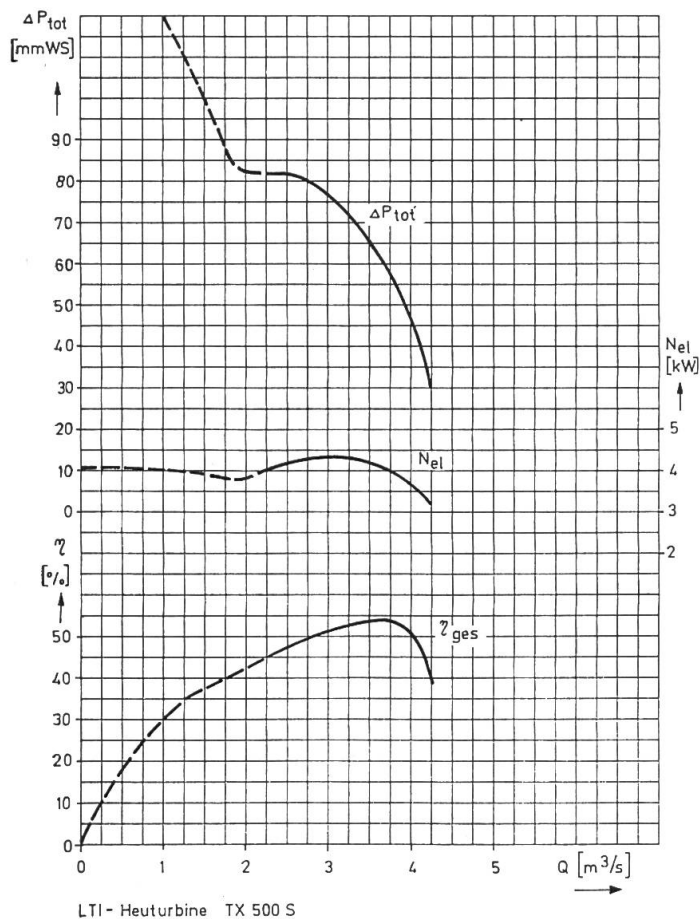
Abb. 5: Ventilator Kennlinien
