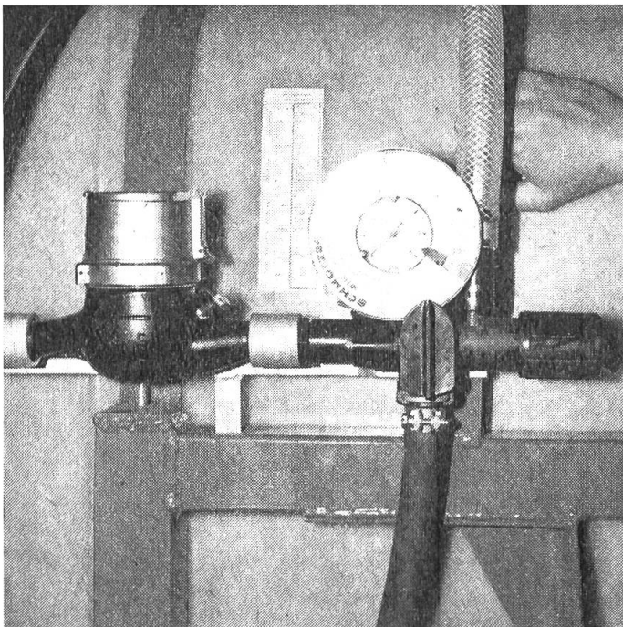
Abb. 4: Am Schmotzer-Dosier-Pilot muss vor Beginn der Arbeit auf einer Aussenskala der von Fahrgeschwindigkeit, Ausbringmenge und Düsendröße abhängige Spritzdruckwert ermittelt und durch eine Kennmarke für die Manometer-Nadel eingestellt werden.
