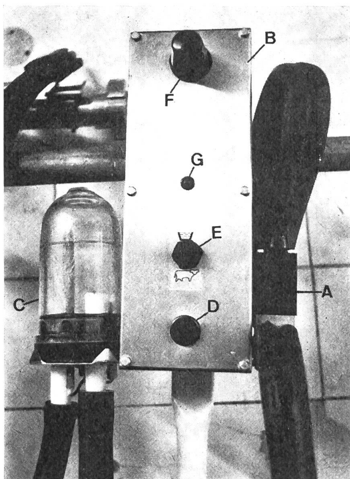
Abb. 8: Miele-«Melkautomatic»
