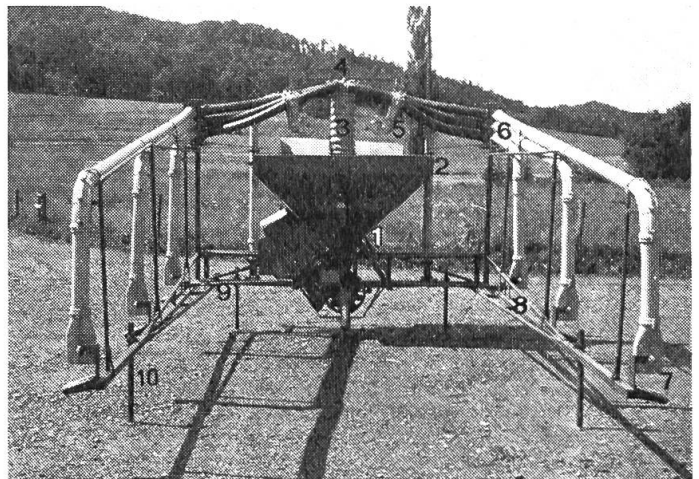
Abb. 1: Pneumatischer Düngerstreuer «Accord PAS» (Transportstellung)
