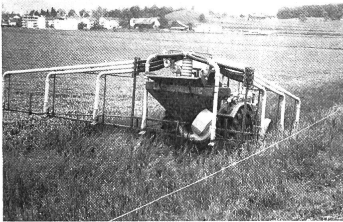
Abb. 7: Einseitiges Streuen am Feldrand. Der rechte Seitenrahmen ist nach vorne geklappt und der Dünger wird über den Sperrschieber mit Umlenkboegen in den Behälter zurückbefördert.
