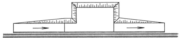
Abb. 6a: Stützmauer und Wandkiesaufschüttung (Grundriss).
