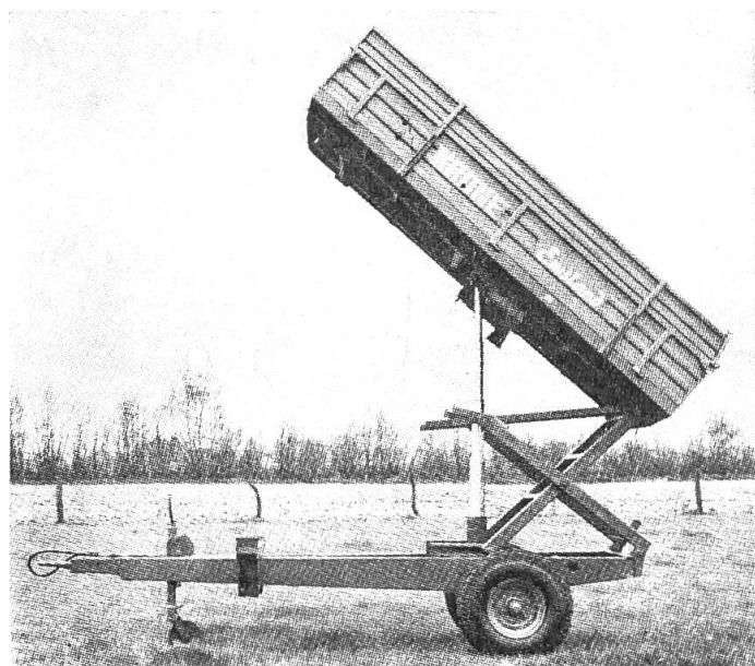
Abb. 4: Hochkipper (Werkbild).
