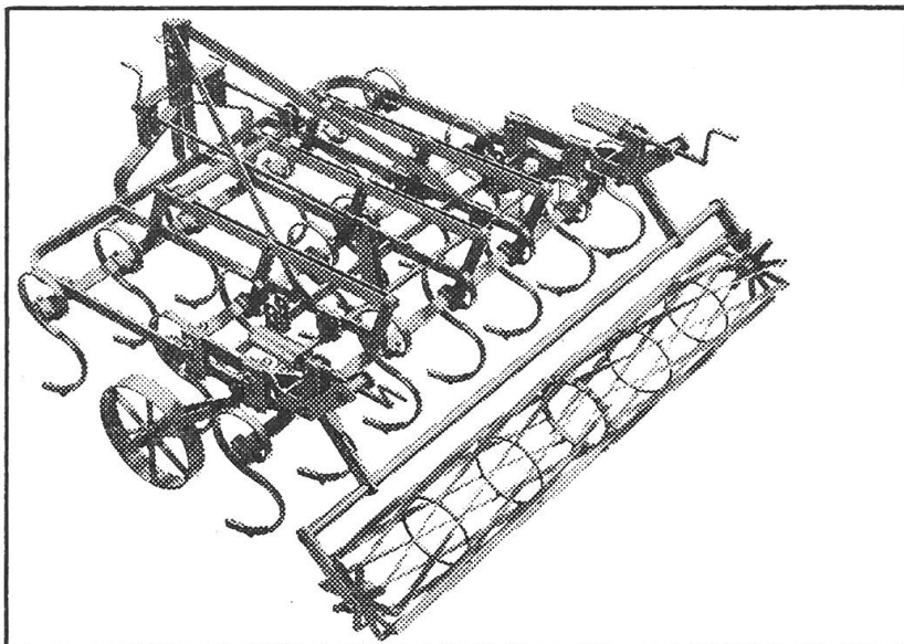
Vibro mit Krümmer Universalgerät für alle Böden; auch zum «Struchen».
