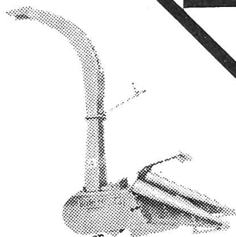
Maishäcksler Hagedorn , dank schnelllaufender Trommel mit 9 Messern 25—30t/h, Exakt- schnitt 4,5 mm, Leistungs- bedarf 30—60 PS, Ge- schwindigkeit 5—8 km/h
