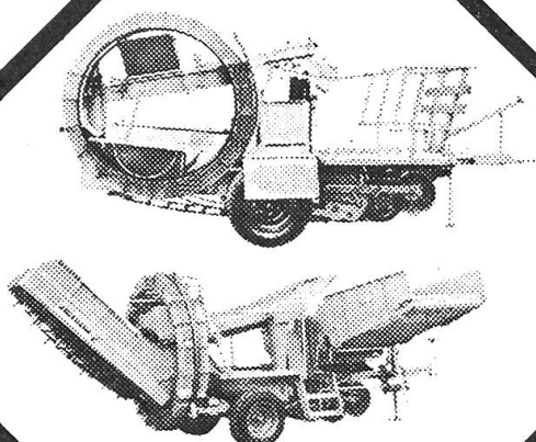
Kartoffelvollernter Wisent , erstaunlich wenig Verlet- zungen!
