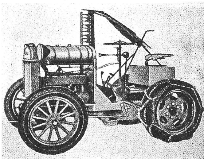
Mafag-Traktor eine Weiterentwicklung des Universal, hergestellt durch die Maschinenfabrik Brugg (heute Maschinen- fabrik Müller AG).
