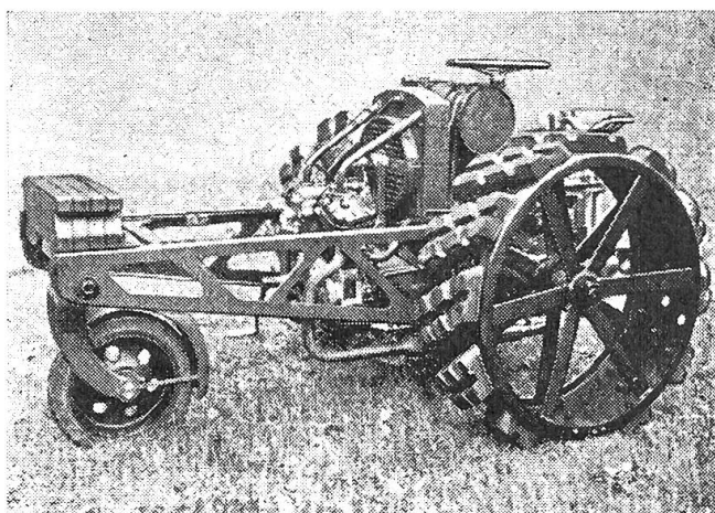
Mafag-Traktor eine Weiterentwicklung des Universal, hergestellt durch die Maschinenfabrik Brugg (heute Maschinen- fabrik Müller AG).
