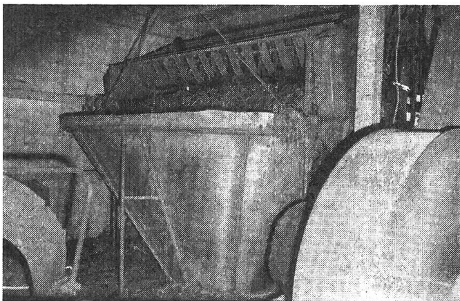
Abb. 5: Gras und Heu werden – von der Dosieranlage kommend – durch den Trichter in die sich darunter drehende Krippe gebracht.
