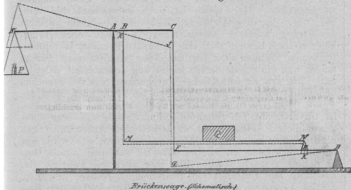
Brückenwage. (schematische)
